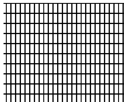
Nr. 4313 mm hole width b x h 1,5 x 3,9 pitch horizontal 2,1 pitch vertical 4,5 opening 62 %
